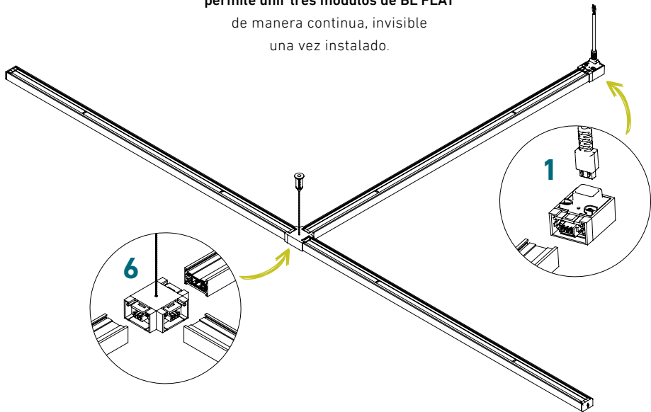
CONECTOR "T" CLAVES BLANCO: P3768-000 NEGRO: P3768-300
