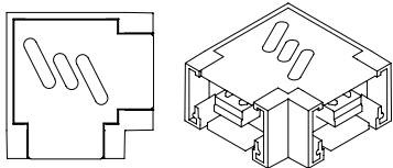
CONECTOR 90° CLAVES BLANCO: P3712-000 NEGRO: P3712-300
