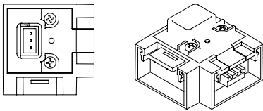
CONECTOR 90° ALIMENTACIÓN VERTICAL TERMINACIÓN CIEGA CLAVES BLANCO: P3759-000 NEGRO: P3759-300
