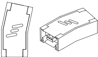
CONECTOR 168° CLAVES BLANCO: P3785-000 NEGRO: P3785-300
