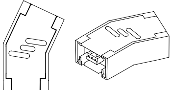
CONECTOR 155° CLAVES BLANCO: P3777-000 NEGRO: P3777-300
