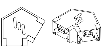
CONECTOR 60° CLAVES BLANCO: P3766-000 NEGRO: P3766-300
