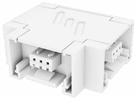
CONECTOR "T" CLAVES BLANCO: P3768-000 NEGRO: P3768-300
