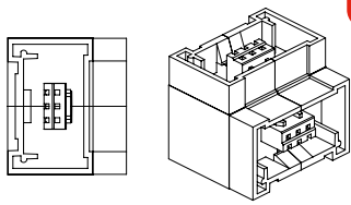
CONECTOR 90° VERTICAL CLAVES BLANCO: P3892-000 NEGRO: P3892-300
