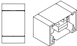
INTERCONECTOR LÍNEA CONTINUA CLAVES BLANCO: P3704-000 NEGRO: P3704-300
